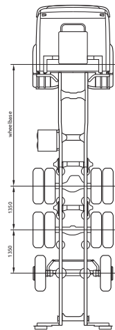
8X4
